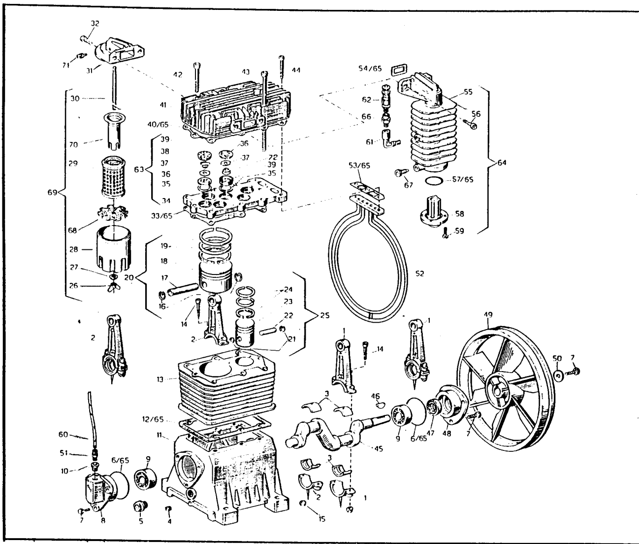
COMPRESSORE (AB 800) / COMPRESSOR (AB 800)
